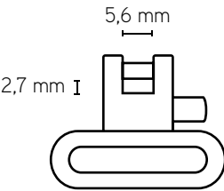
Sling fastening with EU standard swivel for rifle Schließung mit EU standard Riemenbügeln für Waffen
